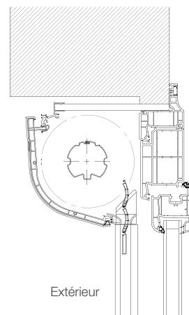
Volet roulant rénovation
