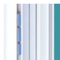
Gâche métallique et condamnation par crémonne multi-points réglables
