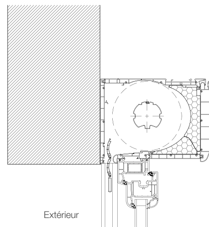
Volet roulant intégré
