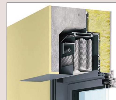
Le bloc-baie BSO ½ linteau
